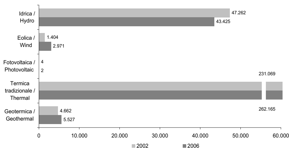
Figura 11.1 Produzione lorda di energia elettrica per fonte energetica utilizzata - Anni 2002 e 2006 (milioni di KWh)
