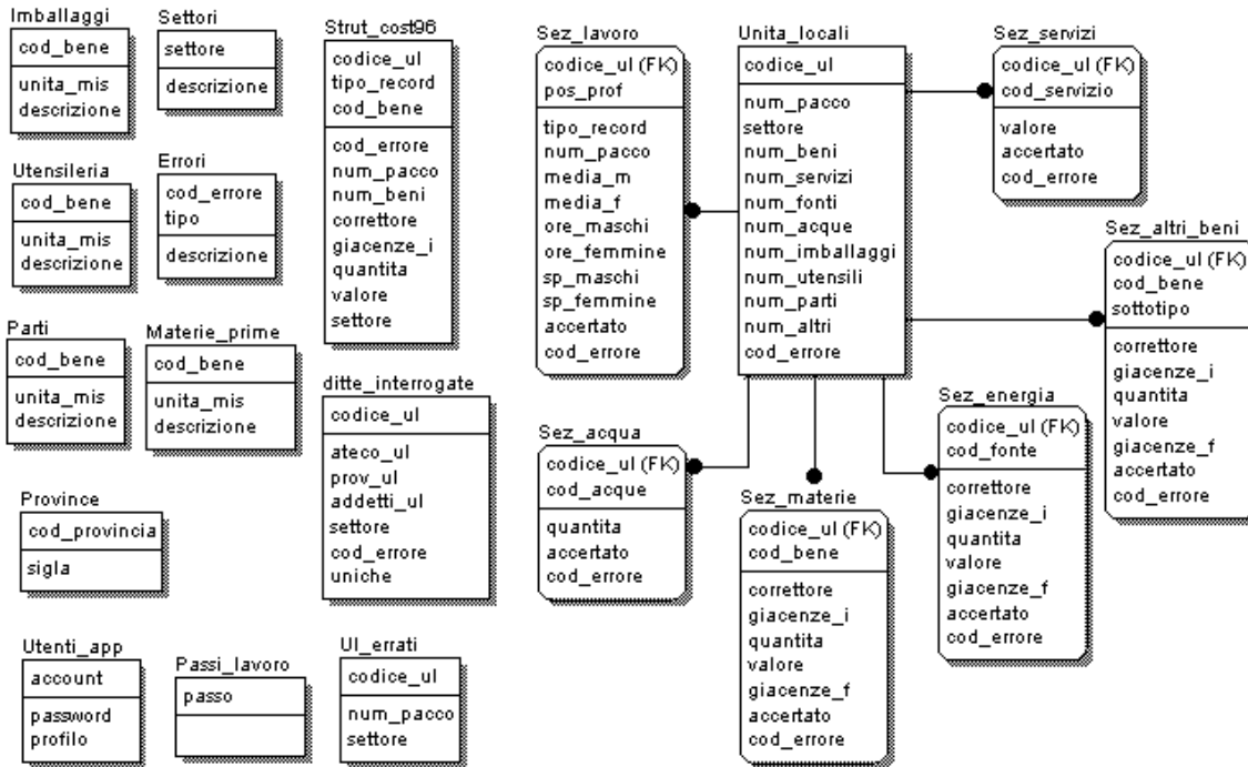
Figura 4-1 : diagramma ER
